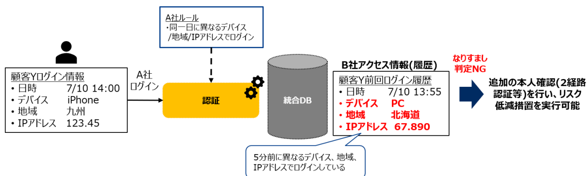
図5-11：統合データ利用による本人認証例
