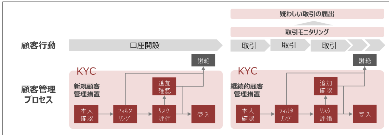
図3-4：KYCプロセス
