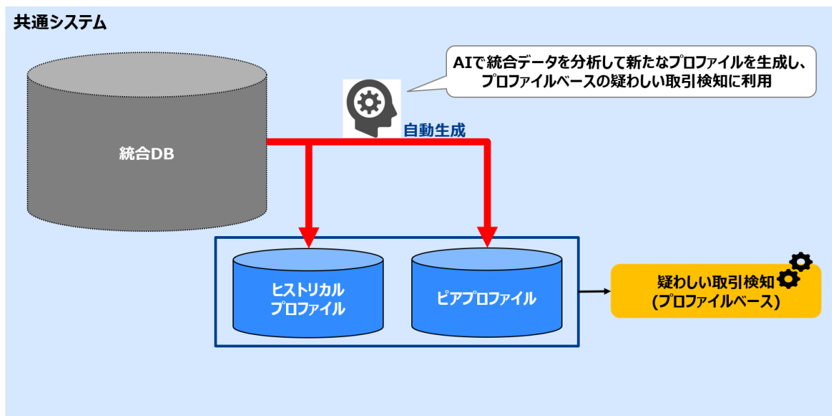
図5-13：統合データの分析による取引モニタリングのプロフィール生成
