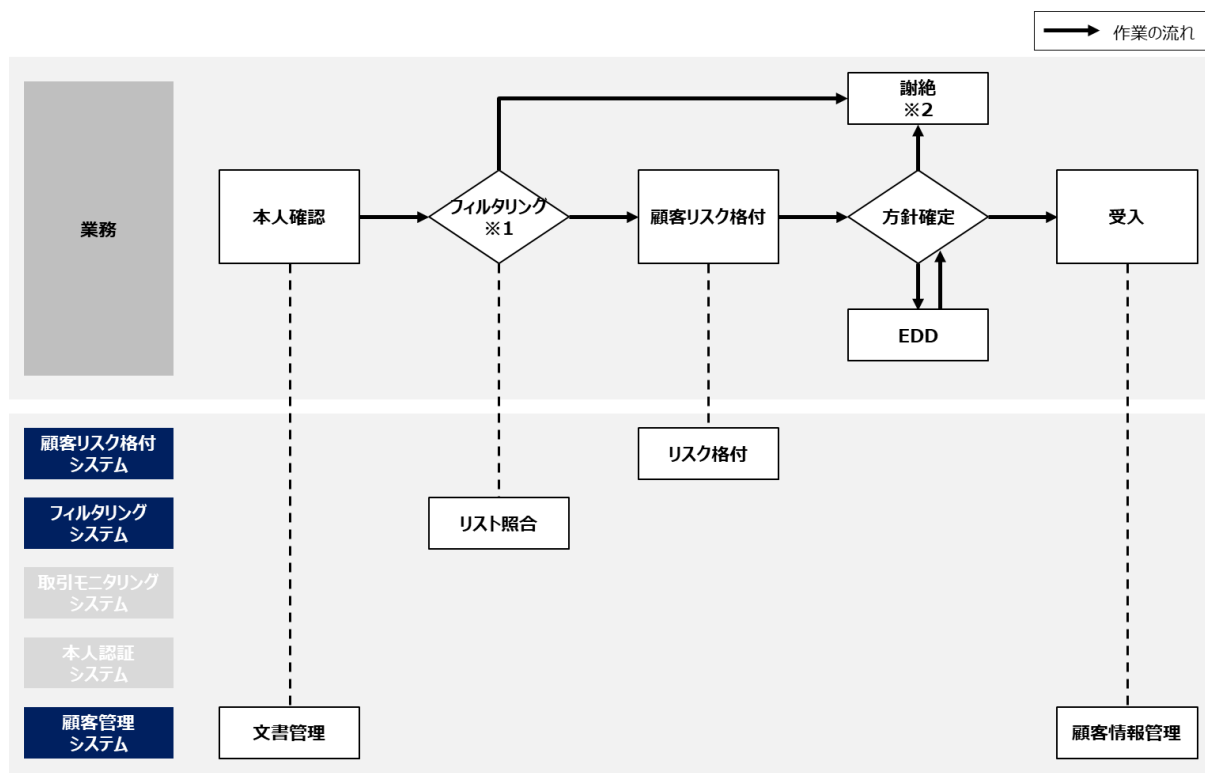
図4-3：新規顧客管理措置の業務プロセスと活用するITシステム例
