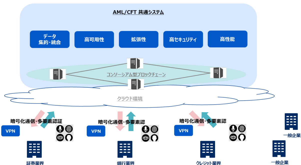
図5-2：共通システムの実現イメージ
