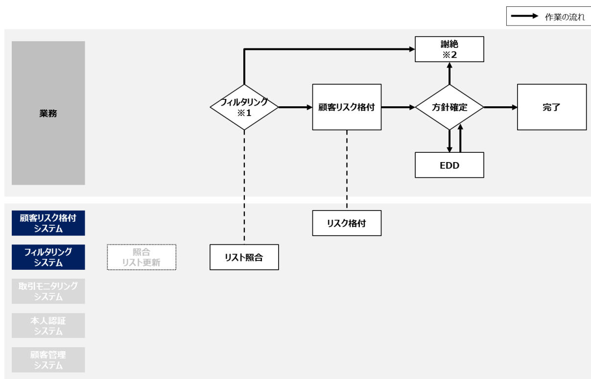
図4-4：フィルタリングの業務プロセスと活用するITシステム例
