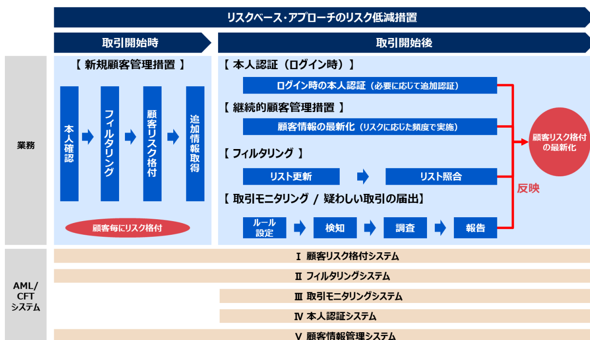
図4-1：リスクベース・アプローチによるAML/CFT業務とITシステム
