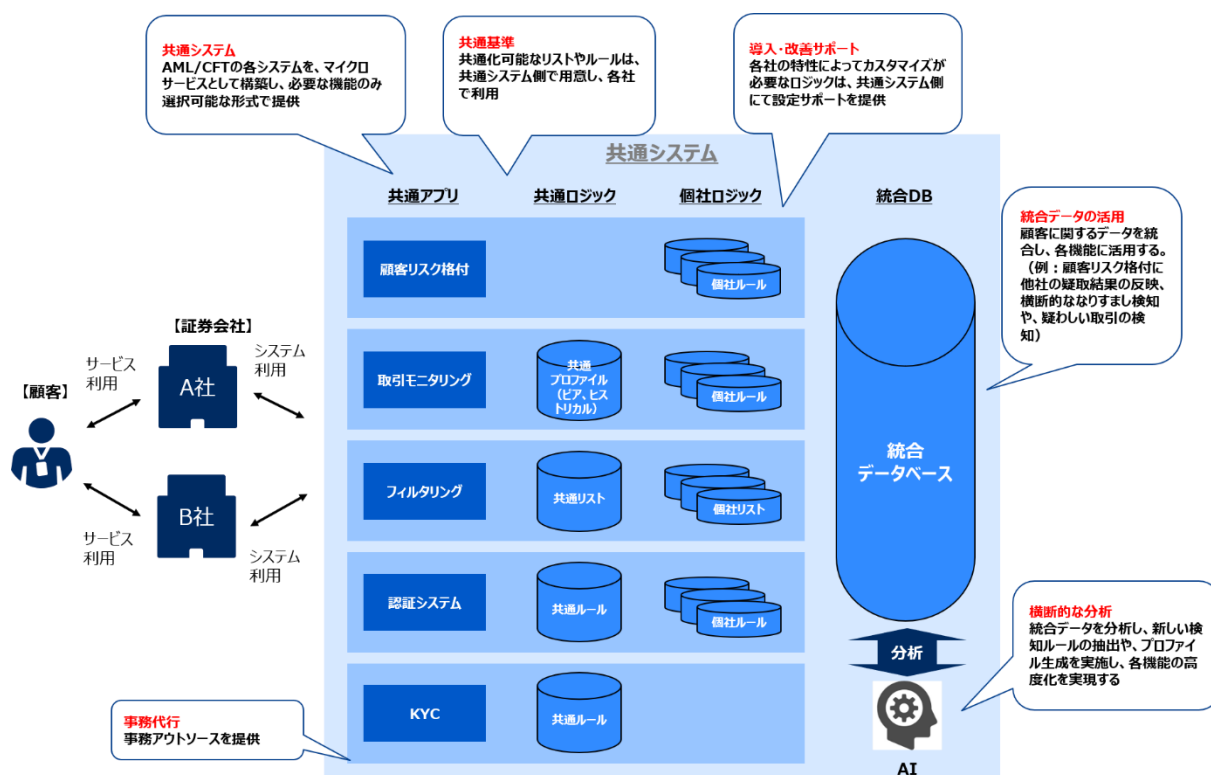
図5-3：共通システムの機能配置例
