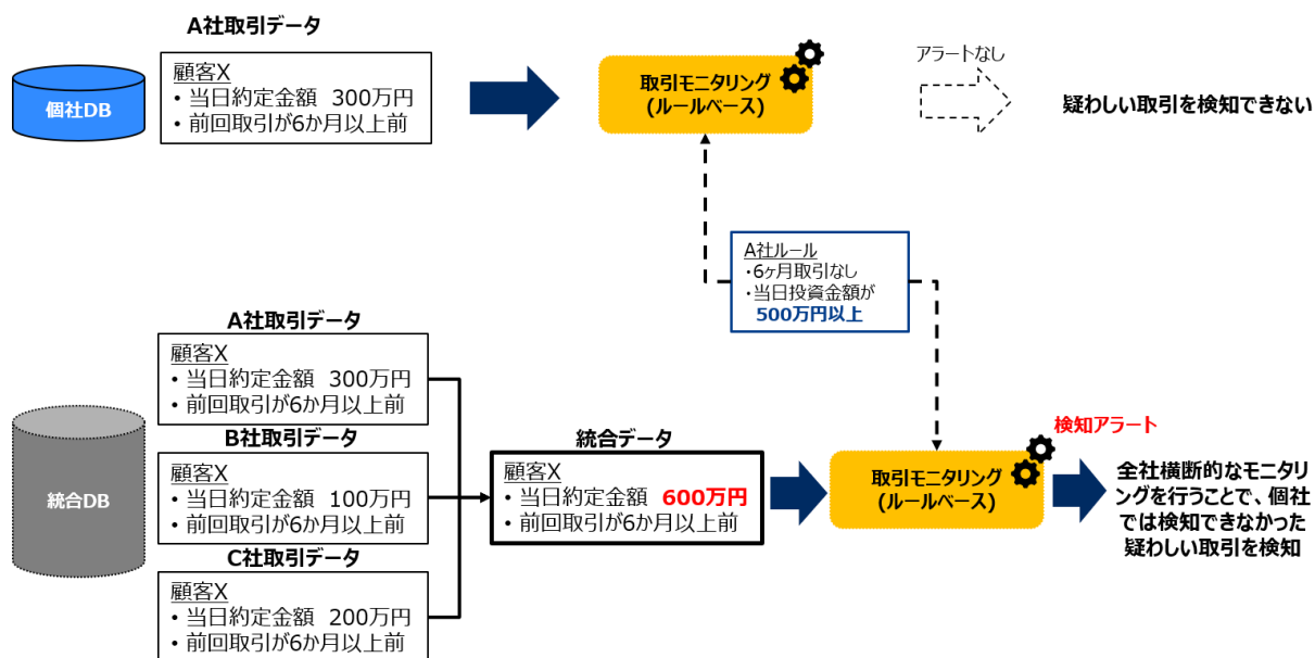
図5-10：統合データ利用による取引モニタリング例
