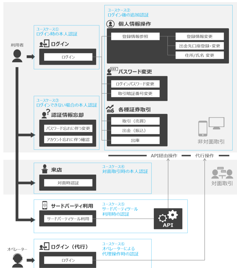
図11：証券サービスにおける本人認証のユースケース
