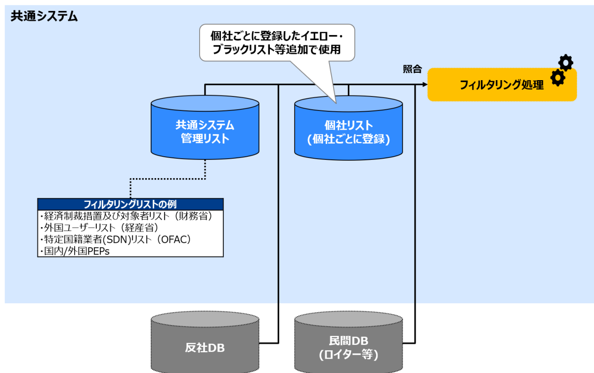
図5-7：フィルタリングのリスト
