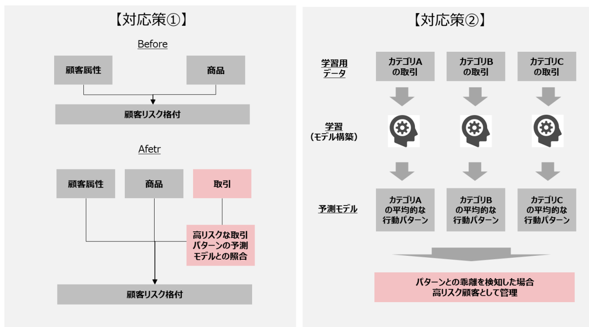
図4-13：顧客リスク格付業務でのAIの活用事例
