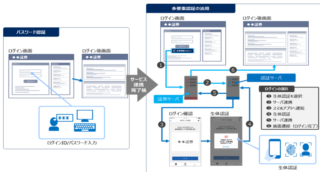
図4-14：多要素認証の活用事例
