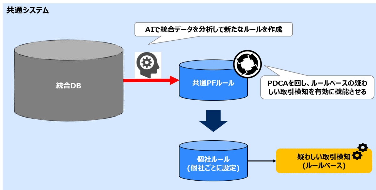
図5-16：統合データの分析による取引モニタリングのルール抽出
