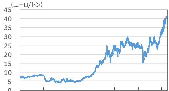
【CO2排出量先物価格（ICE）】
