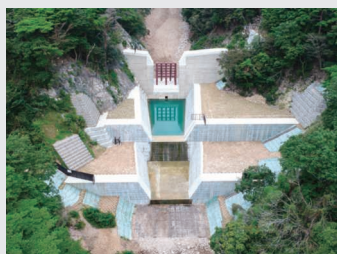
堰堤（えんてい）工事
