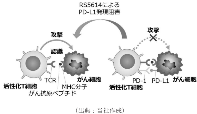
＜図表14 RS5614の免疫チェックポイント分子阻害作用＞
