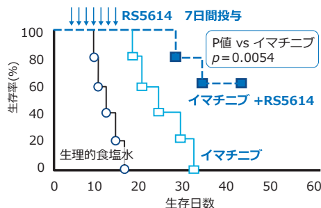
CMLモデルにおけるTKIとRS5614の治療効果
