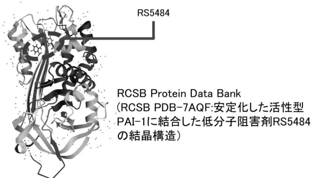
< 図表10 PAI-1とPAI-1阻害薬RS5484複体のX線構造解析 >
