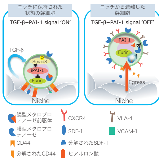
RS5614 (PAI-1阻害薬) の作用機序
